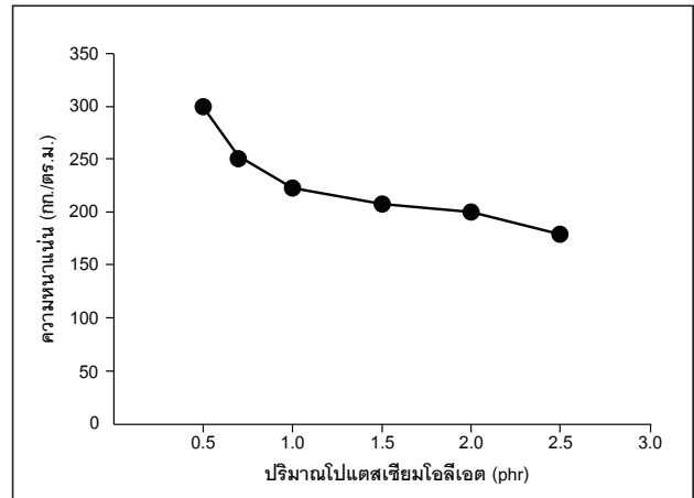
ภาพที่ 1 ความสัมพันธ์ระหว่างปริมาณสารก่อฟอง (โปแตสเซียม โอลิเอต) ที่เติมลงในน้ำยางเพื่อทำให้เกิดฟองโดยใช้เครื่องตีฟอง กับความหนาแน่นของยางพองน้ำ
