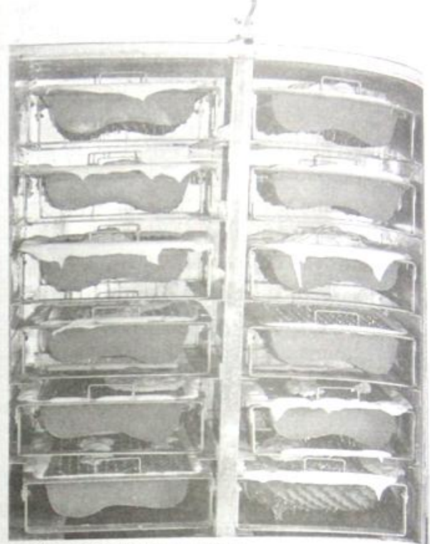
เตาแห้งหมอนยางพารา ขนาด 12 อัน
